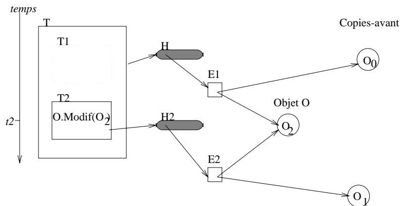
Fig. 5.3 : Les listes d'intention associées à une transaction emboîtée
