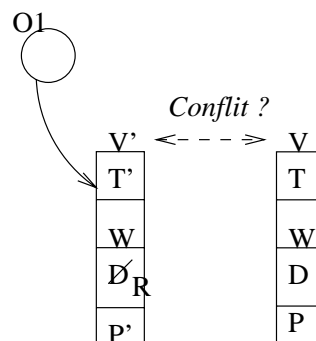
Fig. 4.4 : L'offre du verrou V' permet la pose de V si T est sous-transaction de T'
