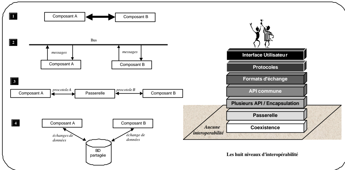
Figure III.15 Les quatre modes et les huit niveaux d'interopérabilité (WfMC – [Verjus et al. 2000, Estublier et Verjus 1999])
