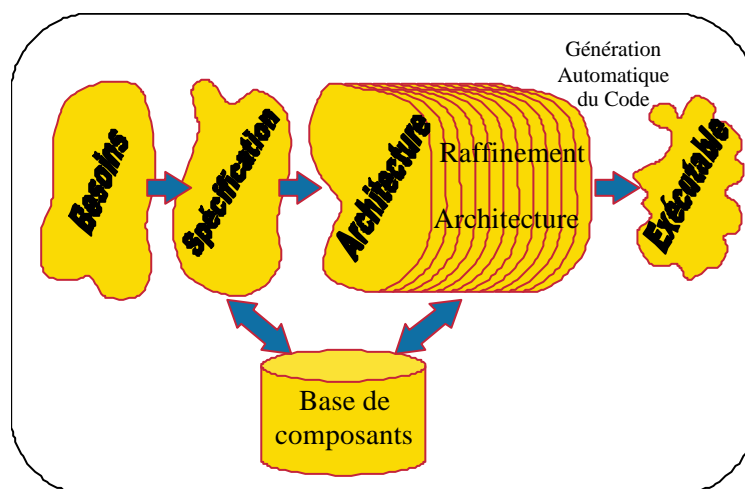
Figure III.4 Processus de développement selon une vision "architecture logicielle"
