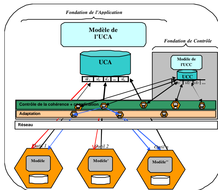
Figure IV.8 Gestion de la concordance
