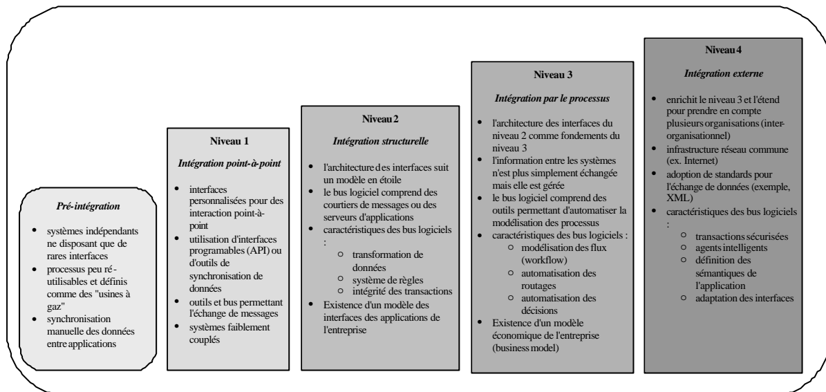
Figure III.11 Modèle de maturité - Intégration d'applications d'après [Schmidt 2000]
