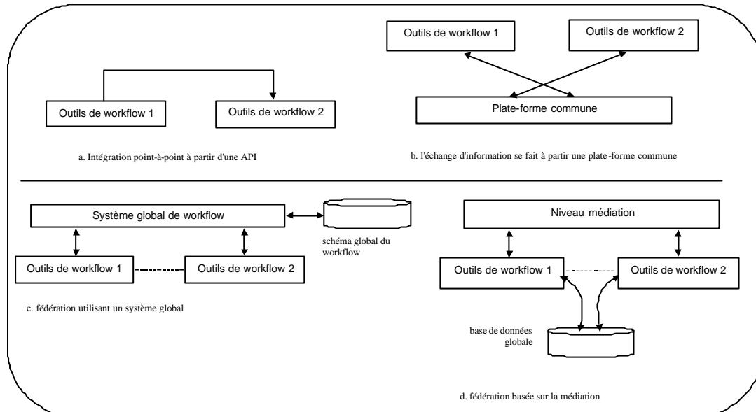
Figure III.26 Différents choix d'architecture pour les fédérations de workflow
