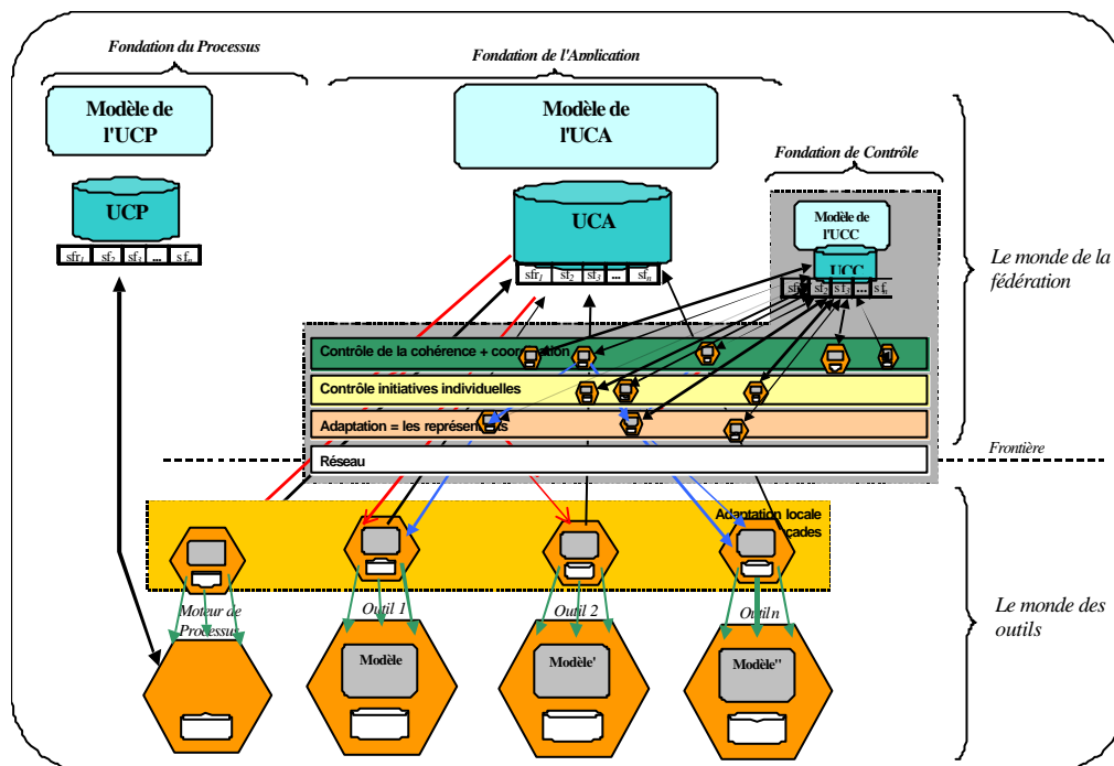
Figure IV.12 Fédération à trois fondations (d'après [Estublier et al. 2001b])
