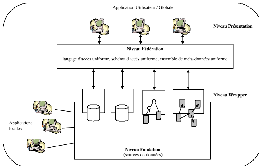
Figure III.24 Architecture pour un système d'information fédéré (d'après [Busse 1999])
