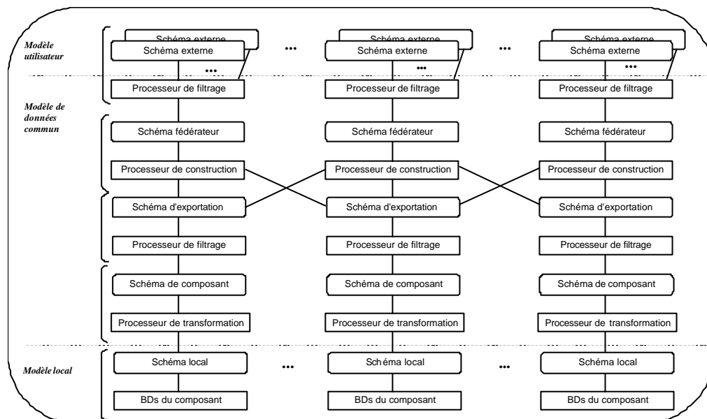
Figure III.25 Architecture du schéma à cinq niveaux (dans [Saltor et al. 1996] d'après [Sheth et Larson 1990])
