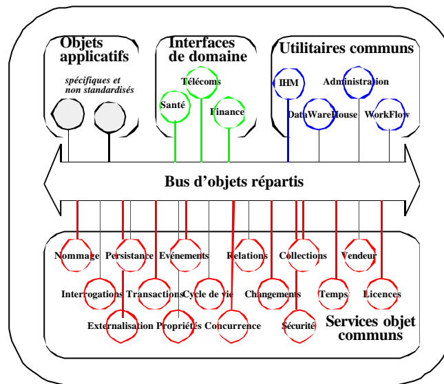
Figure III.2 Architecture de l'environnement CORBA (ou AMO – Object Management Architecture)
