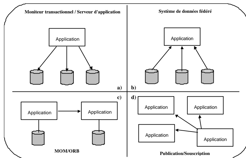
Figure III.13 Modèle opérationnel associé à chacune des approches [Stonebraker 1999]
