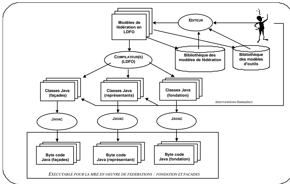
Figure VI.2 La création des exécutables pour la mise en oeuvre d'une fédération avec assistance
