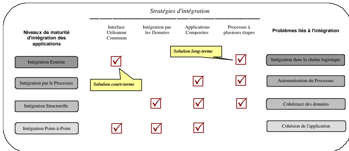
Figure III.12 Plusieurs stratégies d'intégration : la question du choix ...
