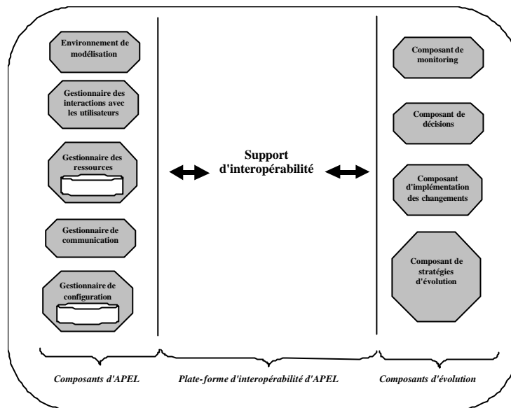
Figure II.4 Architecture de l'environnement PIE (d'après [Amiour et Estublier 1998b])
