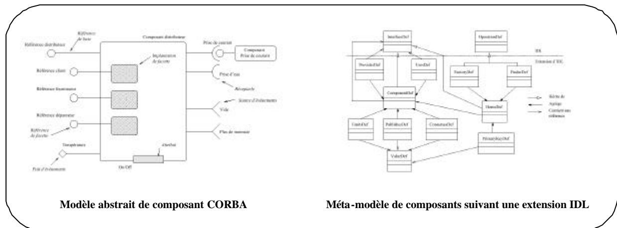
Figure III.3 Modèle abstrait de composant CORBA [Marvie 1999]
